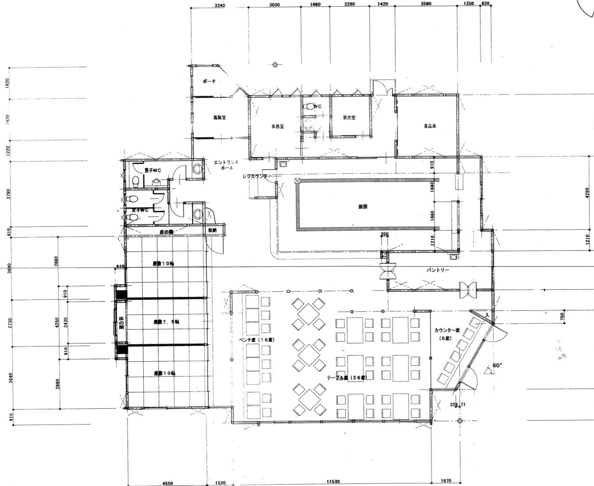
平面図 S=1/100
