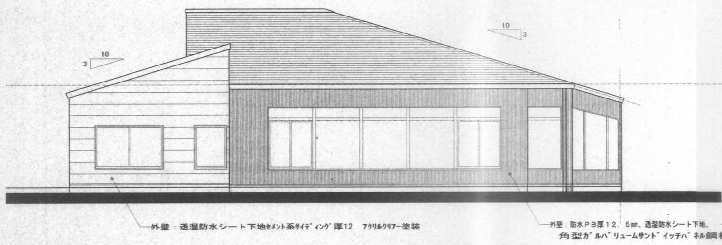
南立面図 S=1/100
